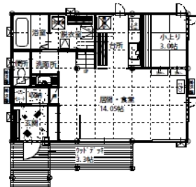
1F平面図
