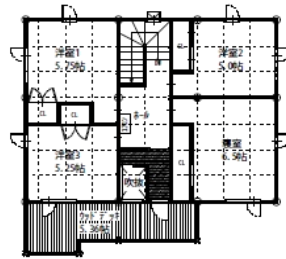
2F平面図
